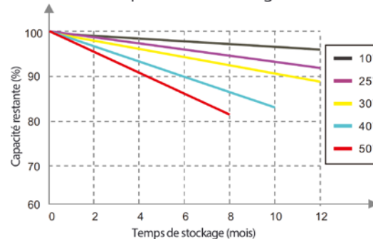
Caractéristiques d'auto-décharge
